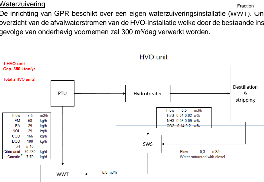
Figuur 6: Schematisch overzicht stappen waterzuivering PTU
