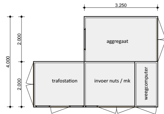
Plattegrond
