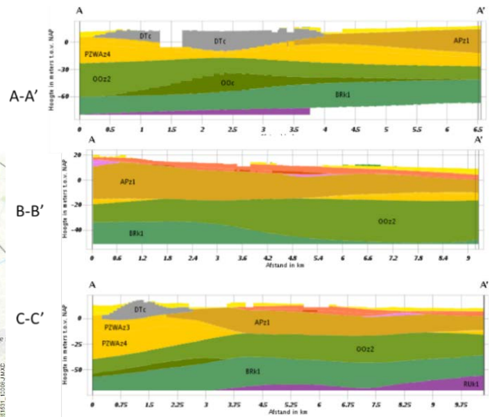
Figuur 2.2 – Dwarsdoorsneden REGIS 2.2 (rechts) inclusief ligging van de dwarsdoorsneden (links)
