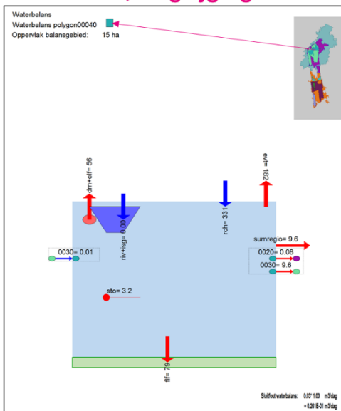
Figuur B5.2 – Waterbalans zones noordzijde Engbertsdijkerven: zones met dikke veenlaag: Links zone 40 (4 m dikke veenlaag), Rechts zone 30 (3 m dikke veenlaag)
