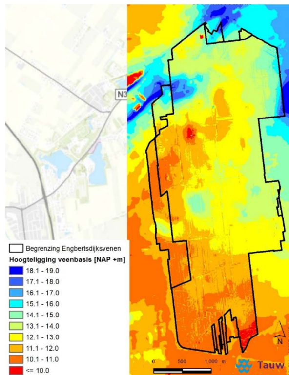
Figuur 2.9 – Berekende hoogteligging veenbasis
