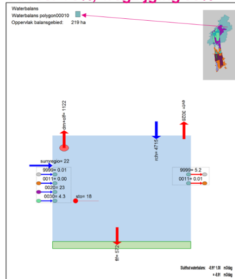
Figuur B5.4 – Waterbalans noordzijde Engbertsdijkvenen; zones met dunner veenlaag: Links zone 20 (2 m dikke veenlaag), Rechts zones 10 (1 m dikke veenlaag)
