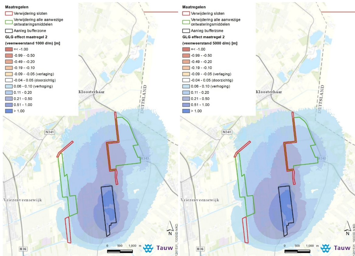
Figuur 6.7 – GLG-verandering in zandlaag als gevolg van bufferzone, bij veenweerstand van 1000 d/m (links) en 5000 d/m (rechts)
